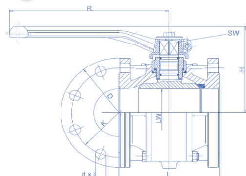
Maßbild mit Option /FA
